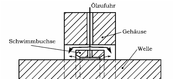
Abb. 1. Prinzipskizze einer Schwimmbuchsenlagerung
